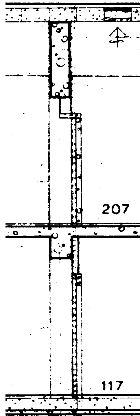
Ensimmäisen ja toisen kerroksen luokkatilojen ja käytävien välisen sisäseinän liittyminen kantaviin rakenteisiin on esitetty poikkileikkauksessa.
