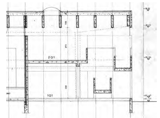
Katoksen, parvekkeen ja kävelyluiskan leikkauspiirustus. Työpiirustus 16 (osa).
