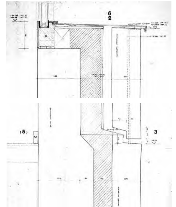
Nauhaikkunan alapuolelle jäävä umpiseinän rakenne. Työpiirustus 117 (osa).
