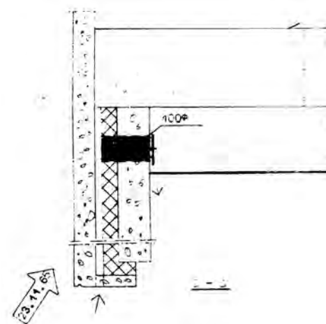
Leikkauspiirustus toisen kerroksen luokkahuoneen korvausilmaelementistä, joka jää piiloon alakaton taakse. Ei mittakaavassa. eCity/Arska: IV6 (osasuurennos).
