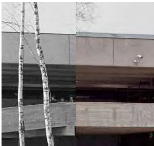
Räystääspellitystä vuonna 1967 (kuvayhdistelmän vasen puoli) sekä vuonna 2013 (kuvan oikea puoli).
