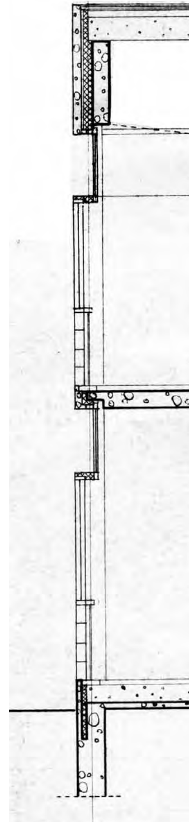
Rakenneleikkaus. Työpiirustus 16 (osa).
