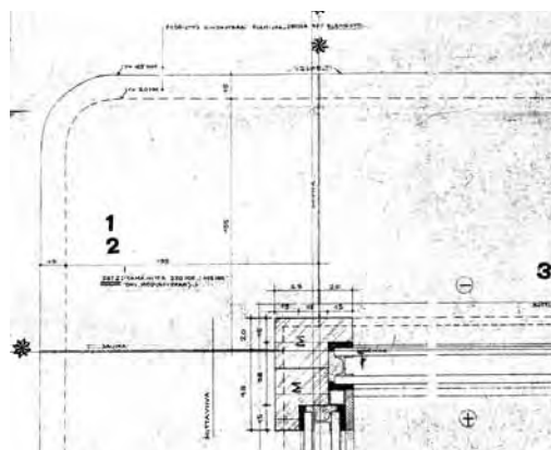
Yläkerran nauhaikkunan pellitystä alhaalta nähtynä. Työpiirustuksen 115 mukaan (ks. alla) pellitys on alun perin suunniteltu noudattamaan betoniseinän muotoa.
