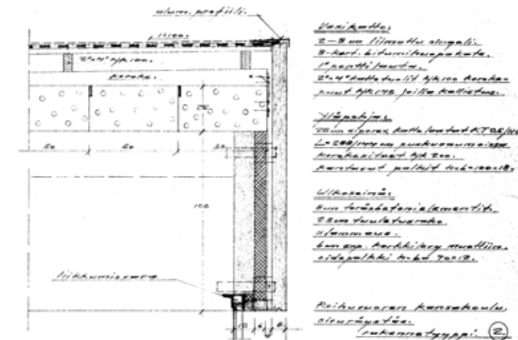
Räystään otsapinnan periaateleikkaus vuodelta 1965. Rakennusselityksen liitepiirros ('rakennustyyppi 2').
