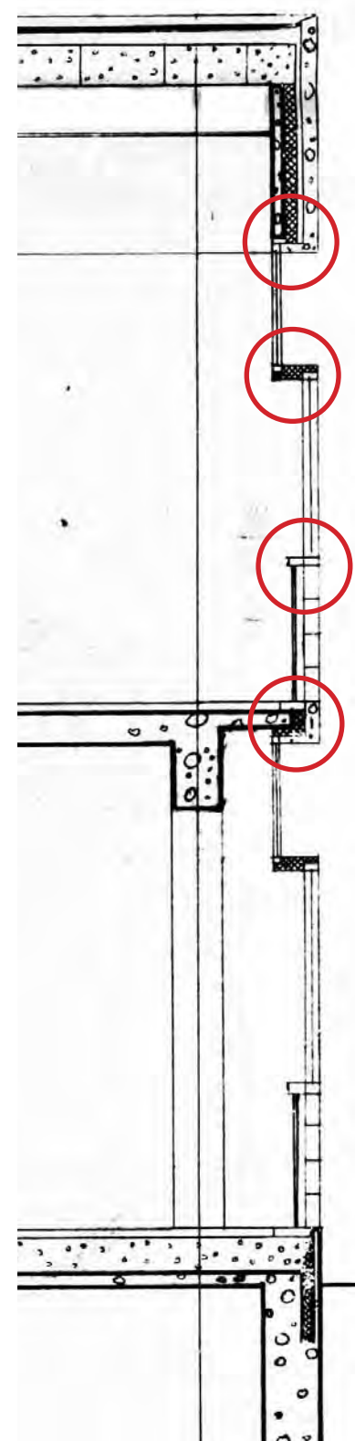
Länsijulkisivun leikkaus; työpiirustus 17 (osa). Piirustukseen on taitossa lisätty neljä punaista ympyrää osoittamaan viereisen detailjipiirustuksen tarkemmin näyttämät kohdat.
