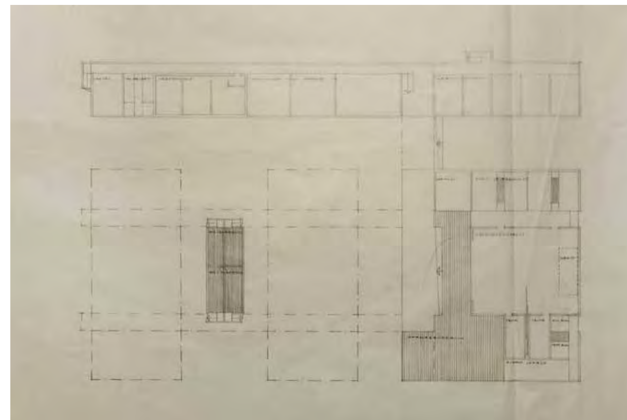
Alempi kerros ja asemapiirustus, 20.6.1962. Ei mittakaavassa. Piirustus: Arkkitehtuurimuseo / Aarno Ruusuvuoren piirustuskokoelma.
