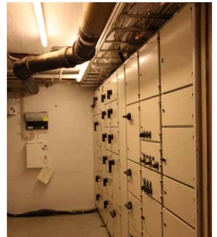
Sähköpääkeskuksen (002) laitteet on uusittu vuoden 1996 sähköremontin yhteydessä.
